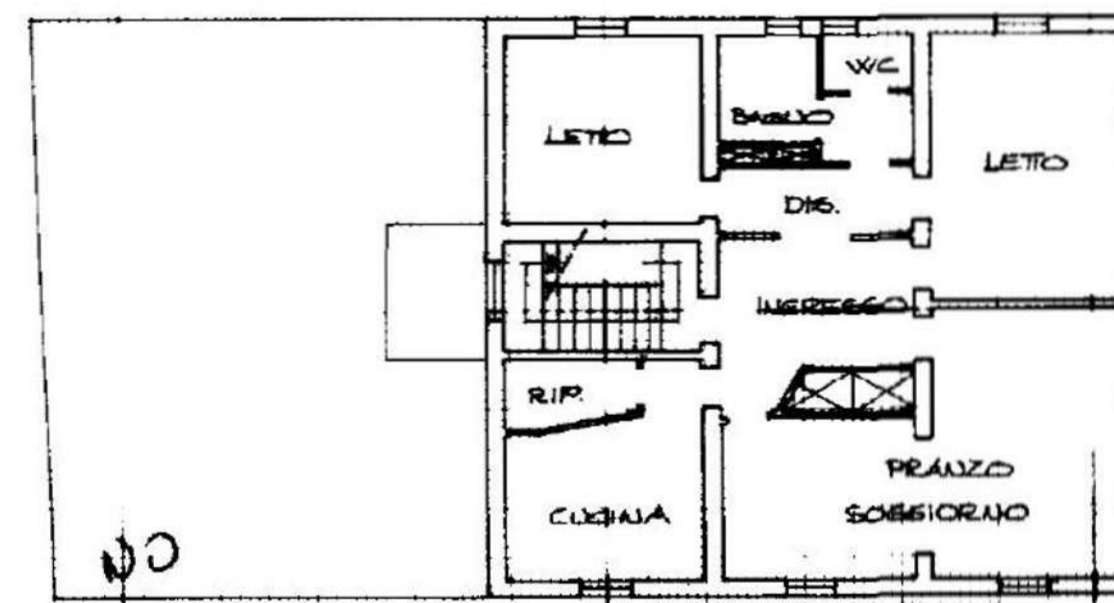
PIANO PRIMO
