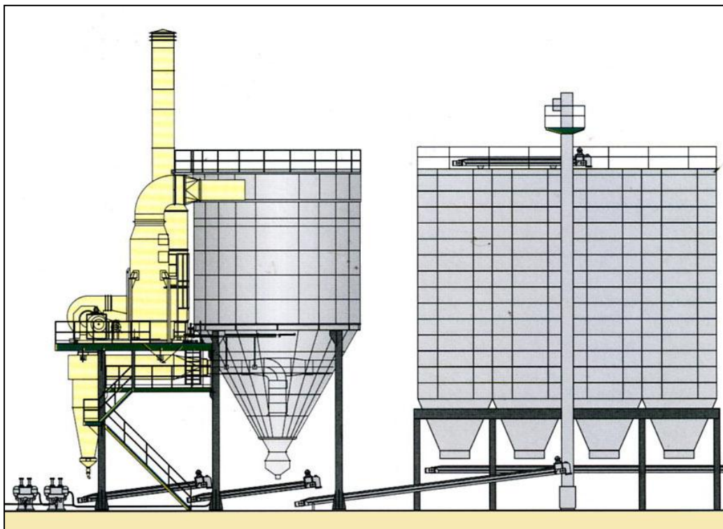
Fig. I.1: schema di apparato per lo stoccaggio di polvere atomizzata
