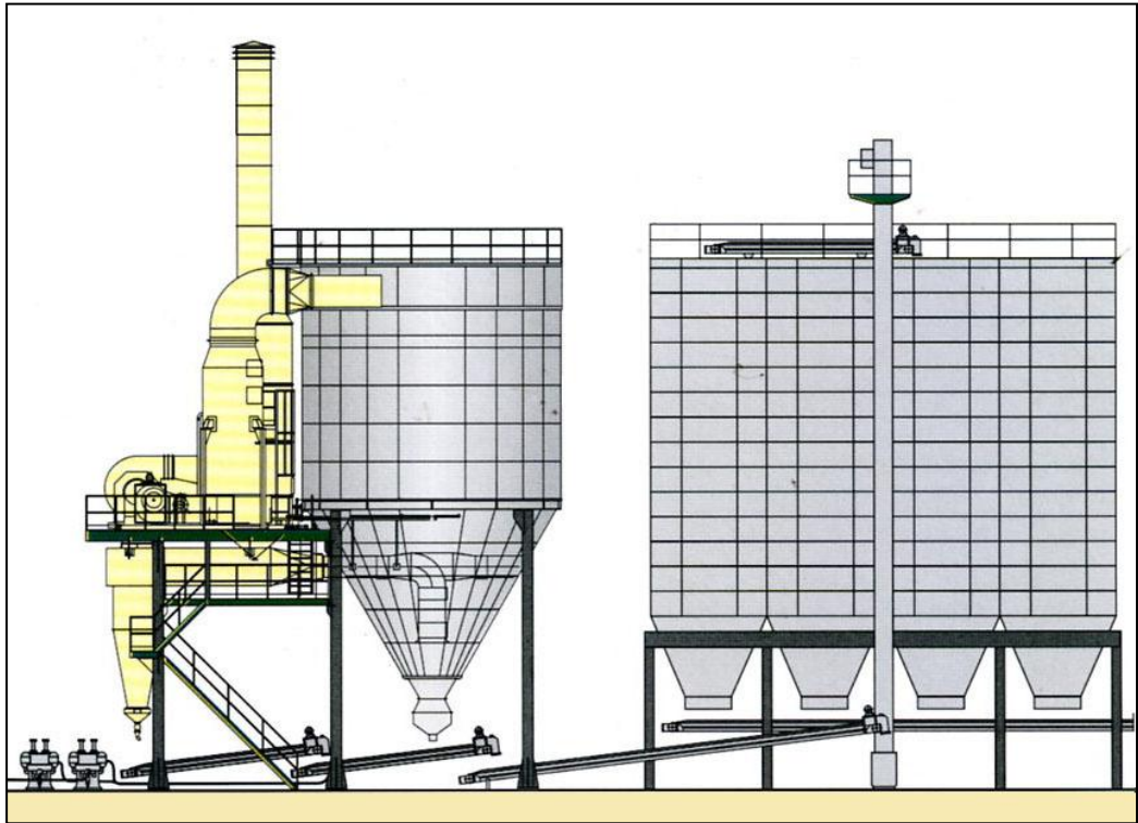
Fig. J.1: schema di apparato per lo stoccaggio di polvere atomizzata
